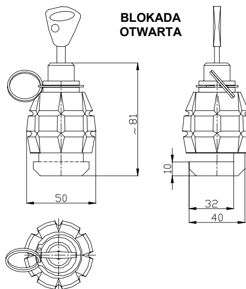
Rysunek złożeniowy blokady motocyklowej:
