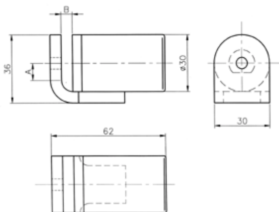
Rysunek złożeniowy blokady motocyklowej:
